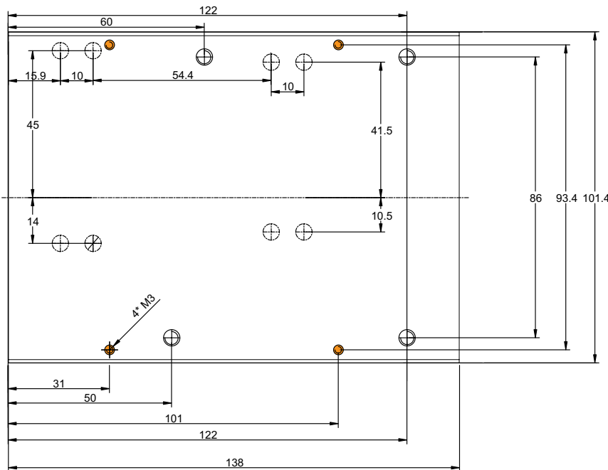
Abmessungen
