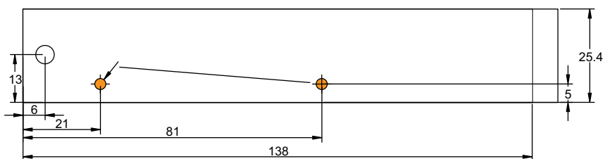
Abmessungen
